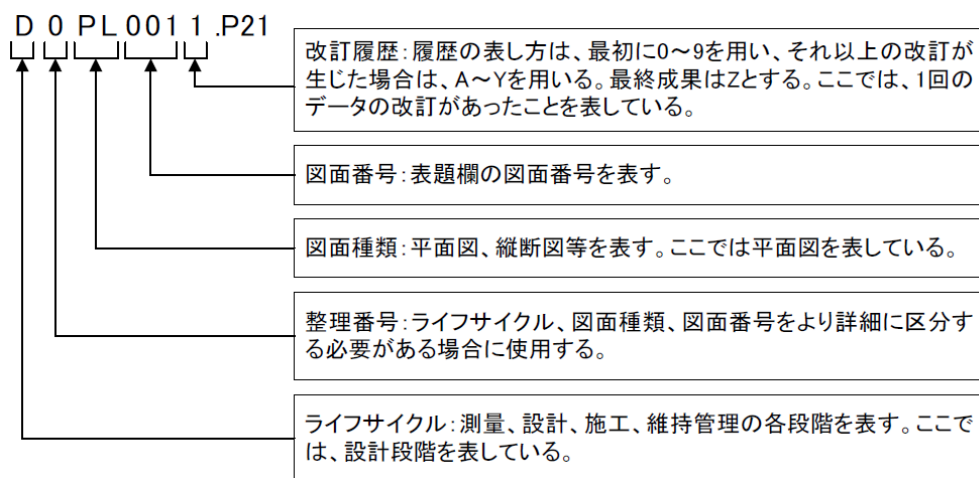
図 2-13 CAD データの命名例
