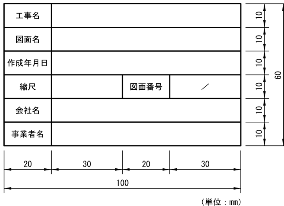
図 4-29 表題欄
