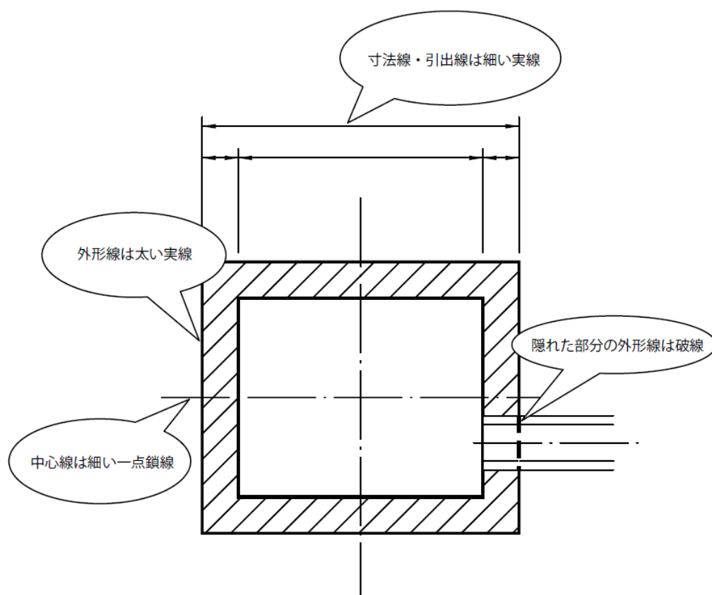
図 2-16 線種と線の太さの利用例
